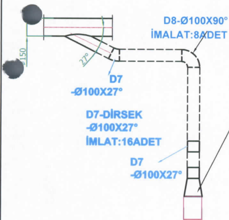
S2 PAKET MAKİNASI ÇIKIŞI VAKUM BAĞLANTI BORUSU ARA PARÇASI İMALAT:8ADET-
