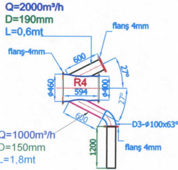
İMALAT:1ADET
