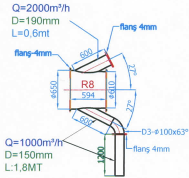
İMALAT:1ADET
