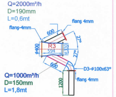
İMALAT:1ADET
