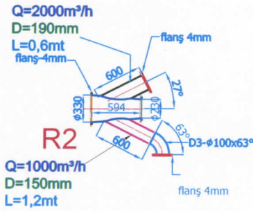
İMALAT:1ADET
