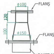
S2 PAKET MAKİNASI ÇIKIŞI VAKUM BAĞLANTI BORUSU ARA PARÇASI İMALAT:8ADET-
