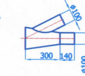
R10- İMALAT:8ADET
