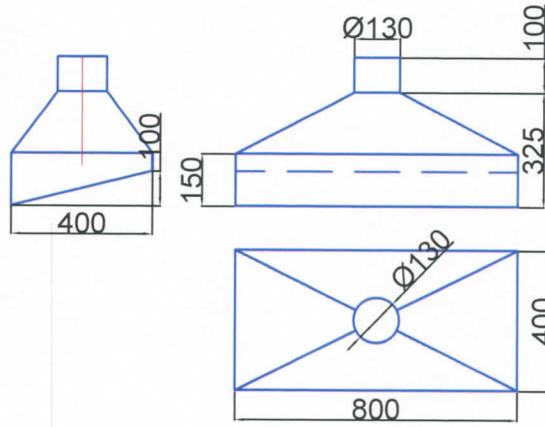
Lif alıcı Kırıcı Davlumbazı imalat:2 adet
