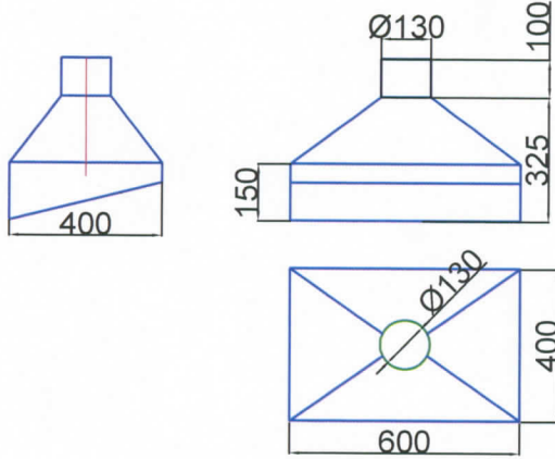
Bant aktarma Davlumbazı imalat:10 adet
