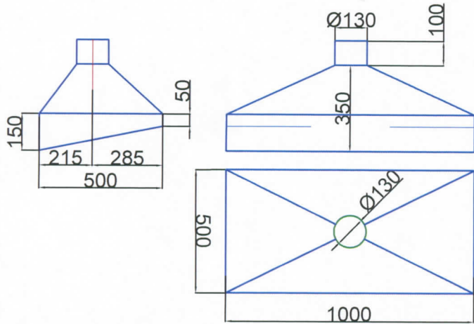
Midilton ve Pakka Davlumbazı imalat:14 adet
