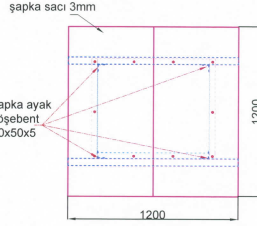
B-B BAKIŞI
