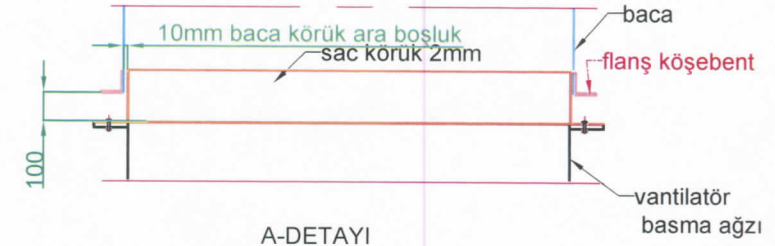
A-DETAYI
